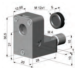
空气吹扫器
