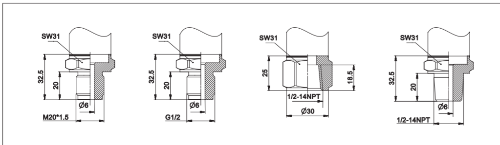
外形尺寸图
